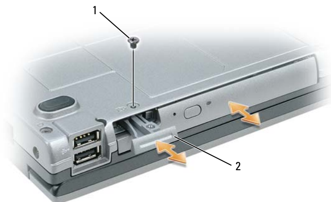
1 Gerätesicherheitsschraube 2 Freigabevorrichtung
