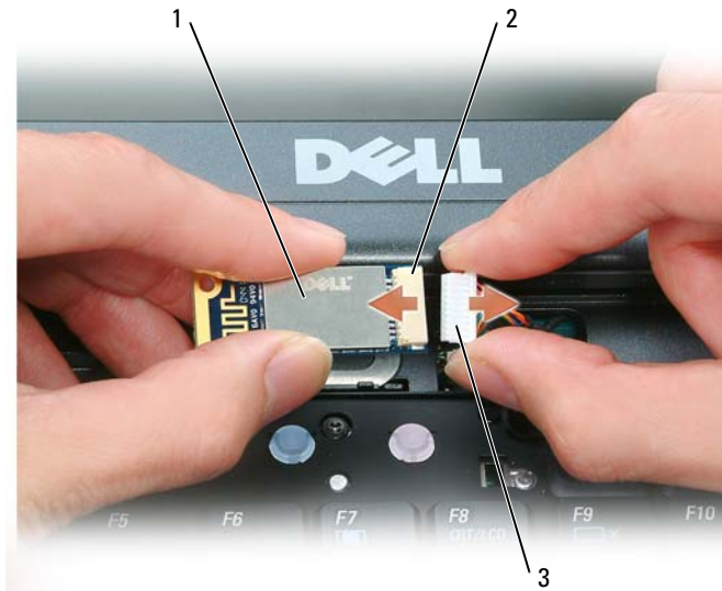
1 Karte 2 Kartenanschluss 3 Kabelstecker
